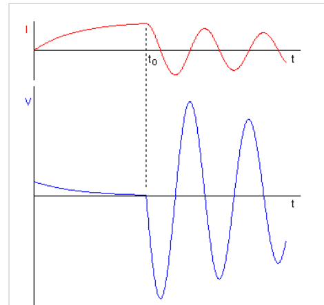
En el instante t_0 el interruptor se abre dejando la inductancia oscilar con las capacidades parásitas.
