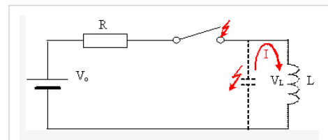
Si la tensión es grande pueden producirse arcos en el interruptor o en la bobina.
